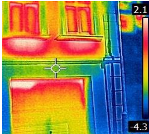
Durch die fehlende Dämmung, ist der Wärmeverlust der Heizkörper unter den Fenstern deutlich zu erkennen.
