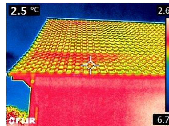
Die Verfärbung des Daches lässt auf eine fehlerhafte Isolierung schließen.
